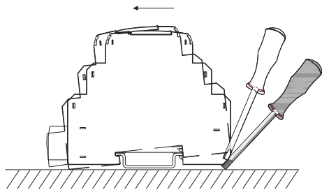
拆卸示意图
